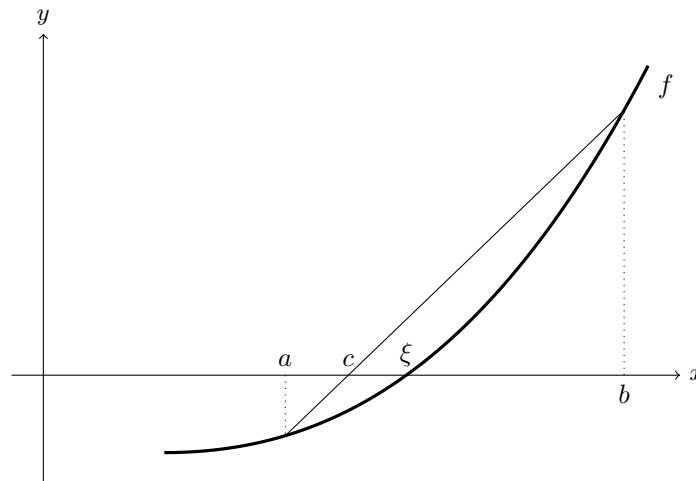
Abbildung 4: Die Regula Falsi berechnet c , die Nullstelle der Verbindungsgeraden, als Näherungswert an die Nullstelle \xi der Funktion f .
