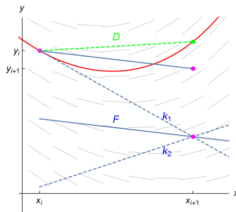
Abbildung 13: Wahl der Verfahrensfunktion F (geometrisch: Fortschritt-Richtung) beim Heun-Verfahren: Mittelwert aus Anfangsrichtung und Richtung am (genäherten) Endpunkt. F nähert den exakten Differenzenquotient ähnlich genau wie das modifizierte Euler-Verfahren D an.
