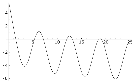
Abbildung 2: Schaubild zur Funktion f(x) = 3 \cos x - \log x . Die Nullstellen von f entsprechen den x -Werten der Schnittpunkte in der Abbildung 1
