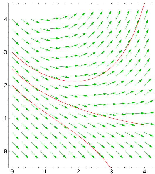
Abbildung 9: Die Differentialgleichung gibt ein Richtungsfeld vor. Drei Lösungen zu verschiedenen Anfangsbedingungen sind eingetragen
